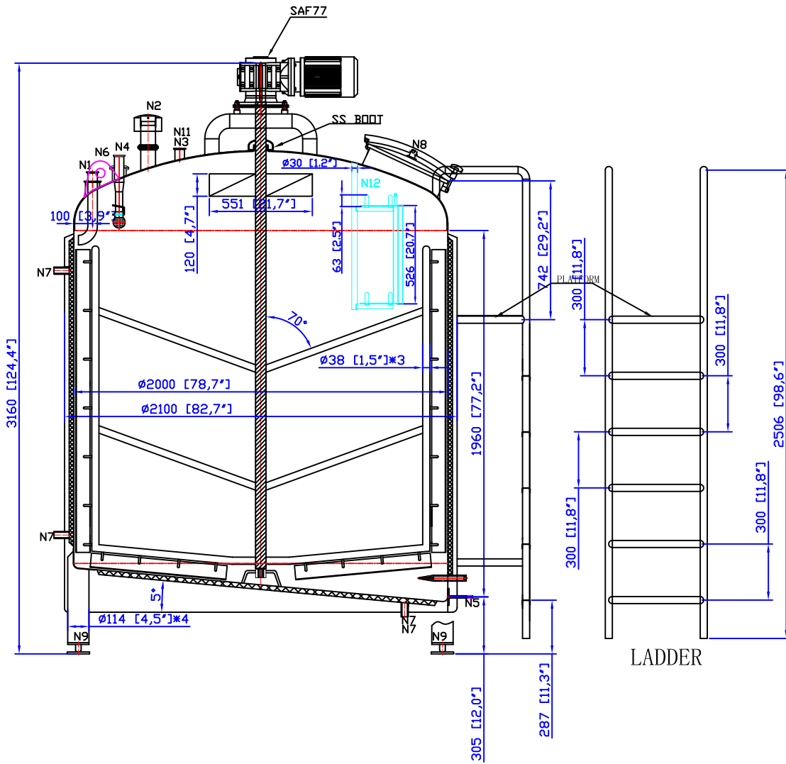
AGITATOR
