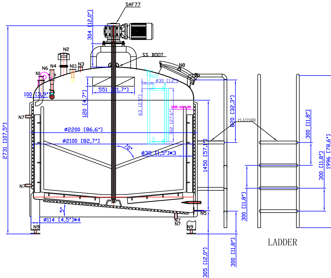
AGITATOR
